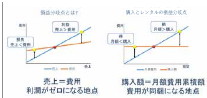
損益分岐点
